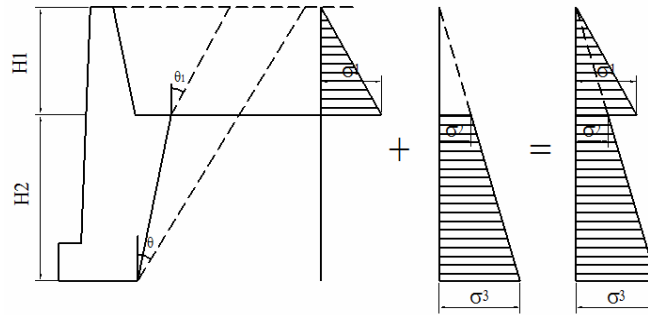
Hình 6. Áp lực đất lên tường chắn có bệ giảm tải
