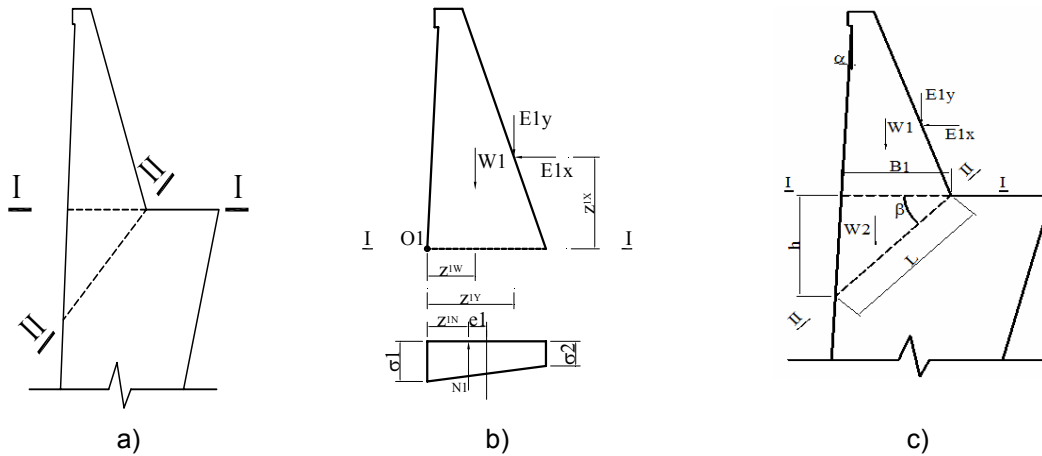
Hình 8. Sơ đồ kiểm toán độ bền các mặt cắt
