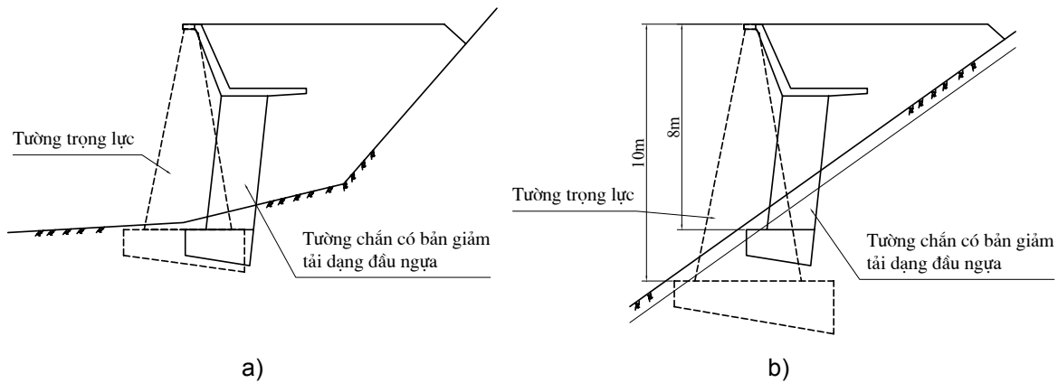
Hình 10. So sánh cùng một chiều cao tường chắn trọng lực và tường chắn có bản giảm tải
