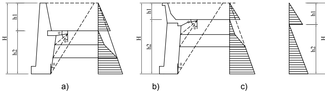
Hình 7. Áp lực đất lên tường chắn có bản giảm tải
