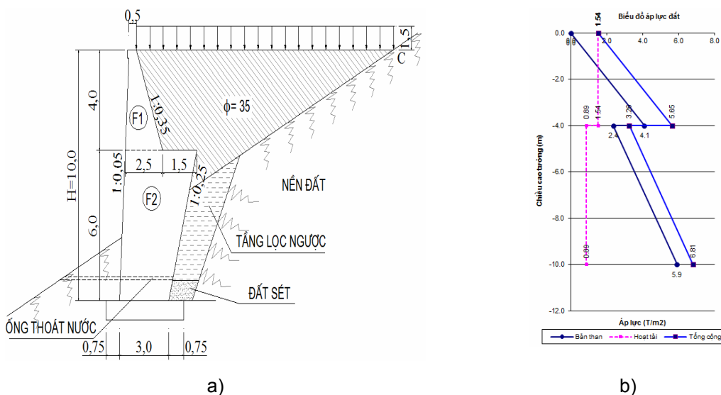
Hình 9. Ví dụ tính toán trong trường hợp cụ thể
