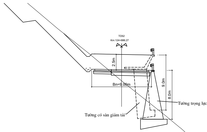
Hình 11. So sánh giải pháp tường chắn có bản giảm tải thay thế tường chắn trọng lực [8]
