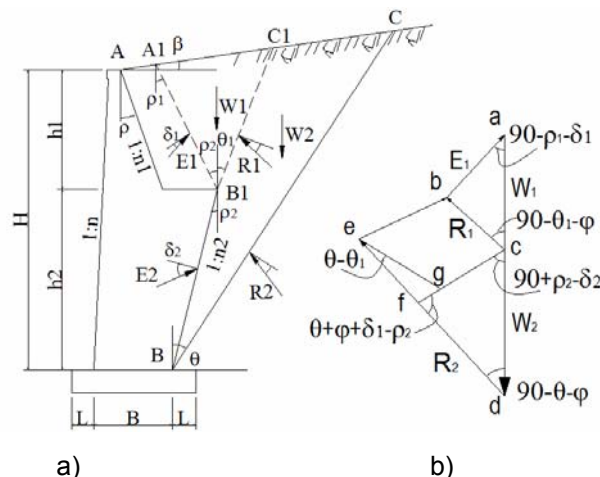
Hình 5. Sơ đồ tính áp lực đất của tường chắn có bộ giảm tải.
