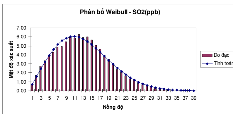
Hình 6. Phân bố Weibull của SO 2
