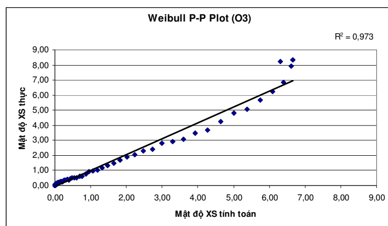
Hình 5. Biểu đồ Weibull P-P Plot của O 3
