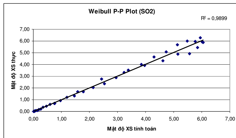
Hình 3. Biểu đồ Weibull P-P Plot của \text{SO}_2
