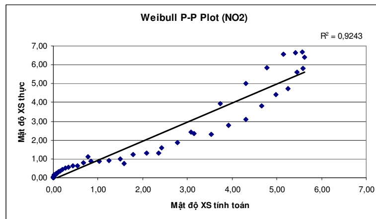
Hình 4. Biểu đồ Weibull P-P Plot của \text{NO}_2
