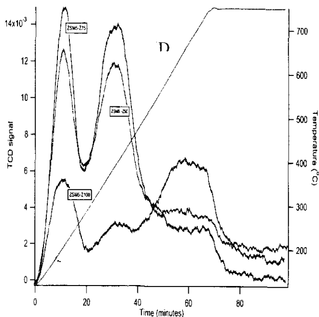
Hình 4: Giảm độ TPD-NH 3 của các mẫu
