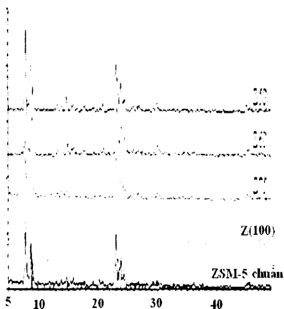
Hình 2: Phổ nhiễu xạ Ronghen của các mẫu
