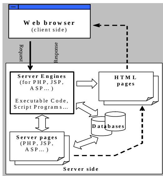
Hình 1. Kiến trúc tổng thể của các ứng dụng Web
