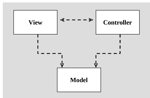
Hình 2. Mô hình tổng thể của mẫu MVC [10, 11]
