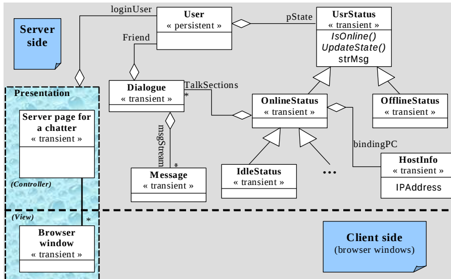
Hình 7. Sơ đồ lớp cho hệ thống quản lý và hiển thị thông điệp được trao đổi trong hệ thống “chat”
