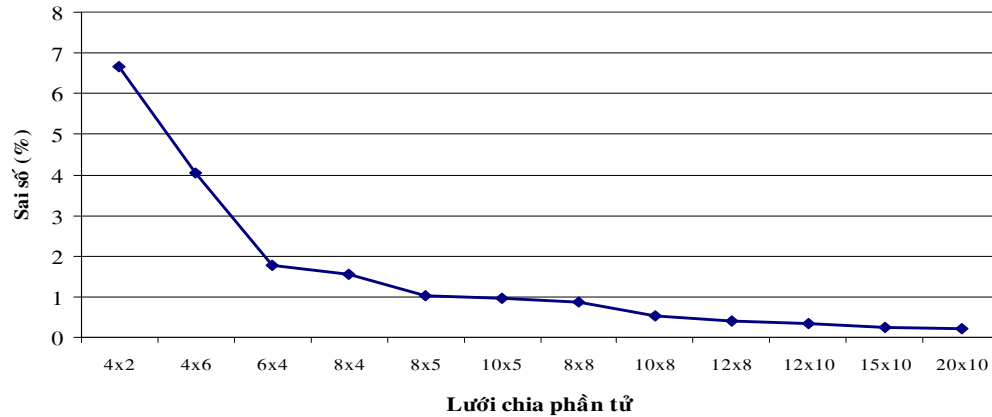
Hình 8. Sai số (%) so với lời giải chính xác của các lưới chia khác nhau.
