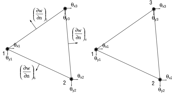
Hình 2. Phần tử HCT sau khi đã giản lược
