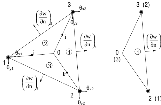
Hình 1. Phần tử tương thích HCT với 12 bậc tự do.
