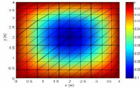
Hình 5. Mode shape của w_{11} và lưới chia 2 \times (10 \times 10) của phần tử HCT (bốn cạnh tựa)
