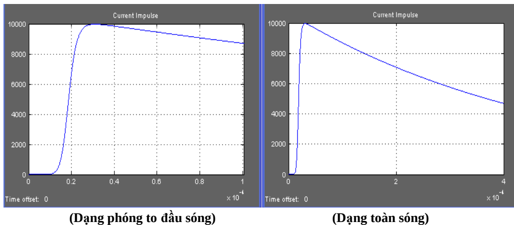
Hình 2. Dạng xung dòng 10kA - 10/350 \mu s
