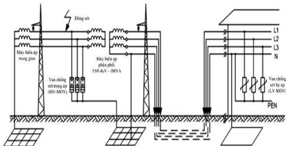
Hình 8. Sơ đồ hệ thống phân phối có trang bị MV-MOV và LV-MOV
