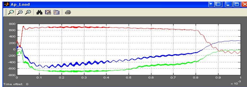
Hình 10. Điện áp trên các pha của tải khi lắp đặt LV-MOV tại đầu cực hạ áp của máy biến áp
