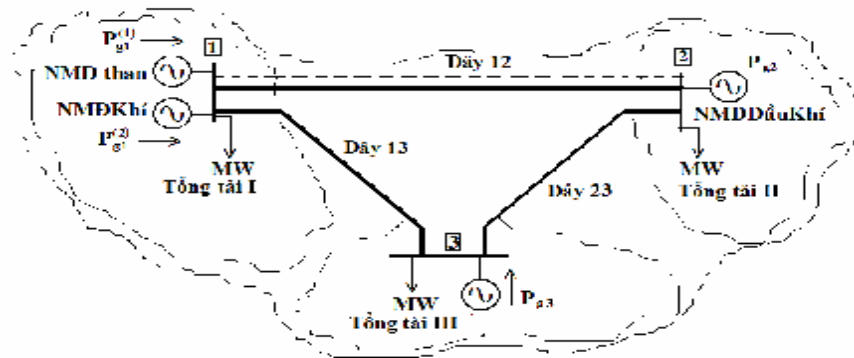
Hình 3 - Sơ đồ phát triển hệ thống giai đoạn quy hoạch từ năm thứ 3 đến năm thứ 6
