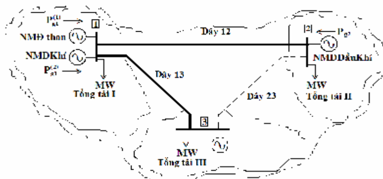
Hình 1 - Sơ đồ khối đầu giai đoạn quy hoạch Hệ thống điện liên kết 3 hệ thống điện khu vực.
