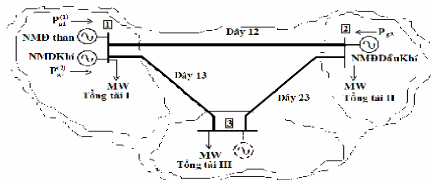
Hình 2 - Sơ đồ phát triển hệ thống giai đoạn quy hoạch từ năm thứ 1 đến năm thứ 3
