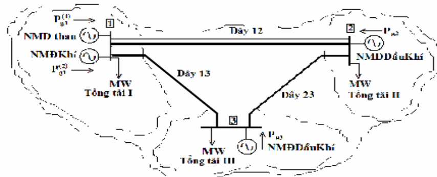
Hình 4 - Sơ đồ phát triển hệ thống giai đoạn quy hoạch từ năm thứ 6 đến năm thứ 9
