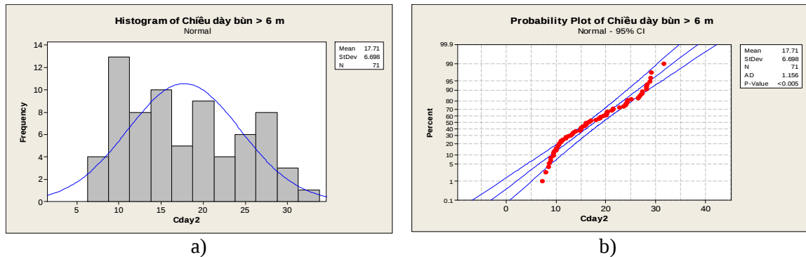
Hình 6. a) Histogram; b) Đồ thị Q-Q plot của nhóm 2
