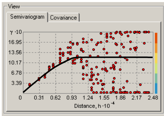
Hình 8. a) Biểu đồ semi-variogram; b) Kết quả nội suy IK
