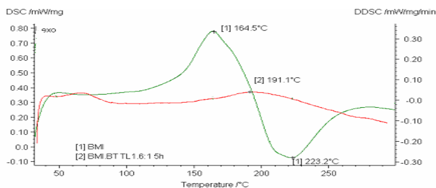
Hình 4. Giải đồ DSC của BMI (đường 1) và BMI.BT. 1,6:1. 5h (đường 2)
