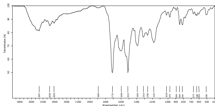
Hình 6. Phổ IR mẫu BMI.BT. 1,6:1. 5h
