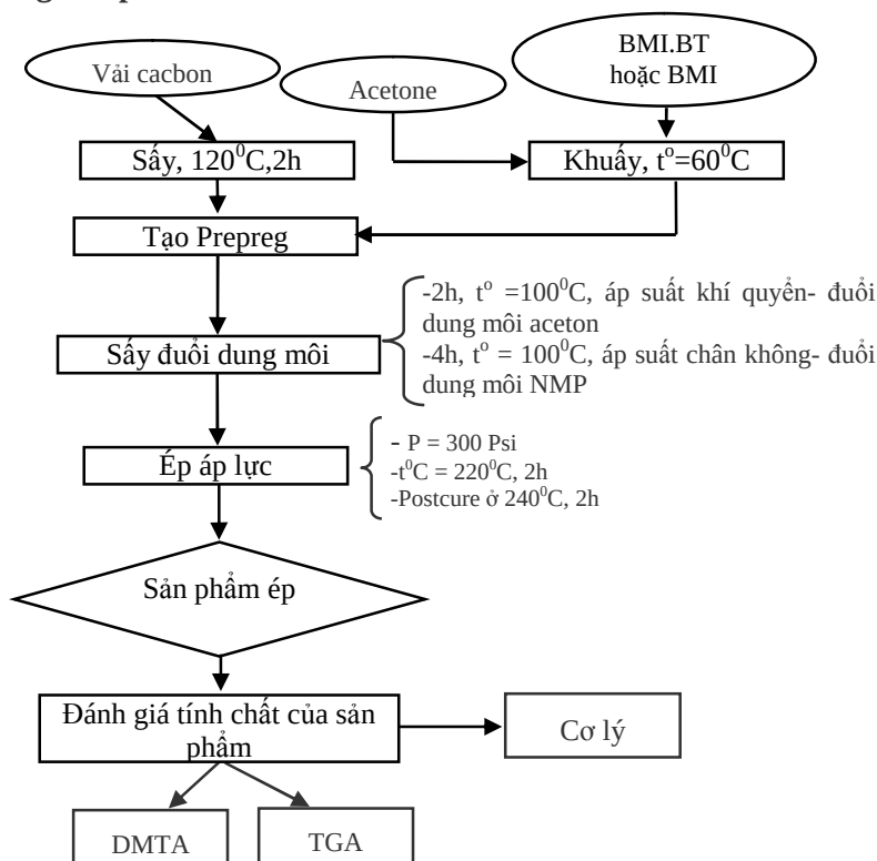
Hình 3. Sơ đồ quá trình gia công composit
