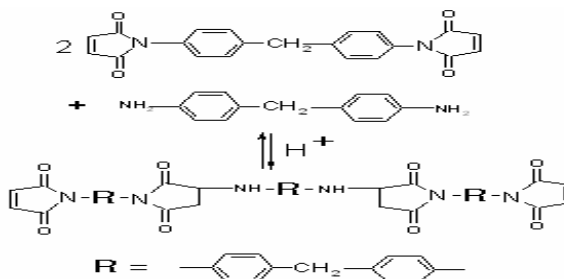
Hình 2. Phản ứng biến tính BMI bằng DDM ở tỉ lệ 2:1 [1]
