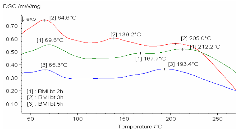
Hình 7. Giải đồ DSC của 3 mẫu biến tính ở tỉ lệ biến tính x=1,6 theo 3 thời gian phản ứng khác nhau
