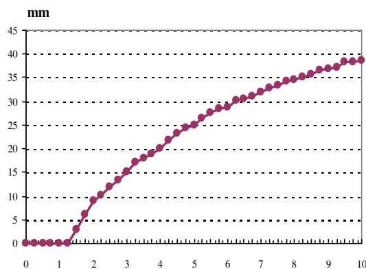
Hình 4a. Bề dày lớp băng trên ống theo thời gian đo từ thực nghiệm
