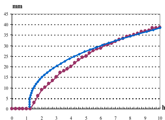
Hình 5b. Sự tương đồng của 2 quá trình tạo băng khi bỏ qua thời gian làm lạnh nước ban đầu
