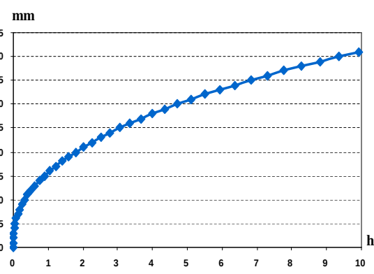
Hình 4b. Bề dày lớp băng trên ống theo thời gian được mô phỏng trên máy tính
