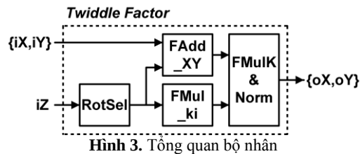
Hình 3. Tổng quan bộ nhân
