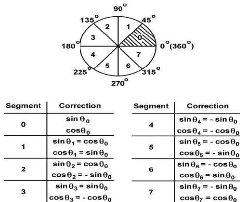
Hình 2. Các góc chuẩn hóa trong vòng tròn lượng giác
