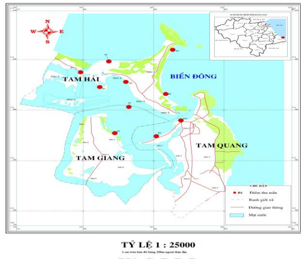
Hình 1. Sơ đồ các điểm thu mẫu
