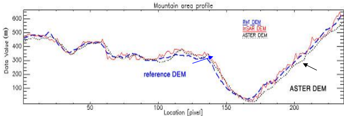
Hình 7b. So sánh cao độ giữa DEM ASTER, DEM INSAR
