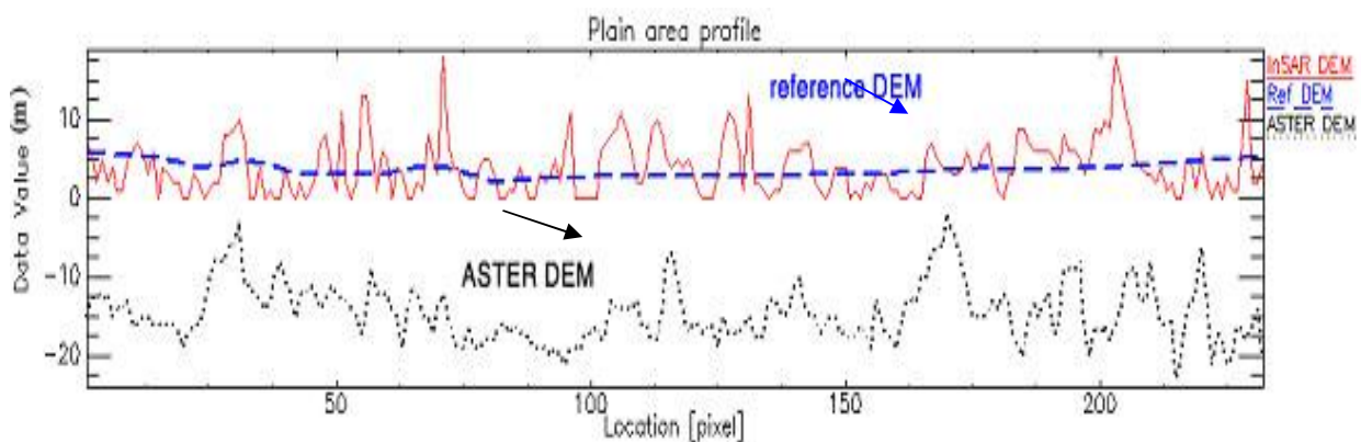
Hình 7a. So sánh cao độ DEM ASTER, DEM INSAR
