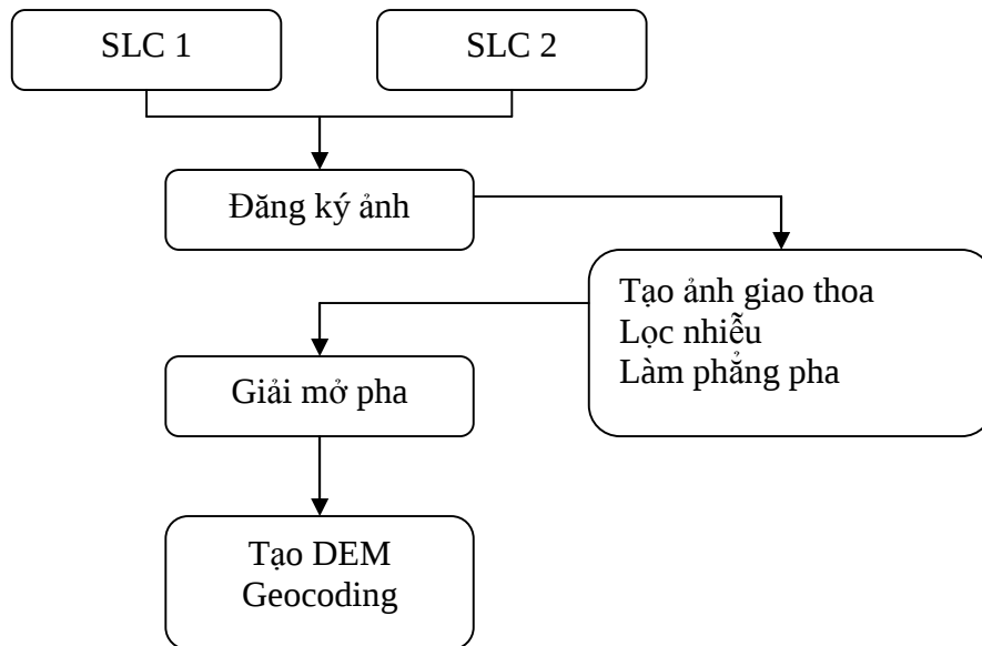
Hình 4. Quy trình xử lý kỹ thuật InSAR
