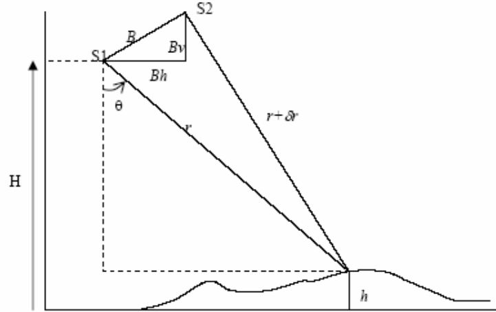
Hình 3. Cấu hình hình học InSAR
