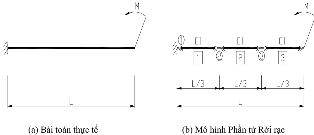
Hình 7. Bài toán dầm console chịu moment tập trung
