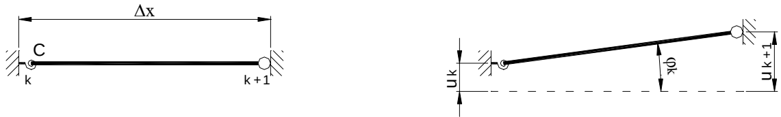
Hình 1. Mô hình phần tử mẫu PTRR sử dụng các biến chuyển vị nút của El Naschie [1]
