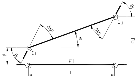
Hình 4. Phần tử Rời rạc biến thể
