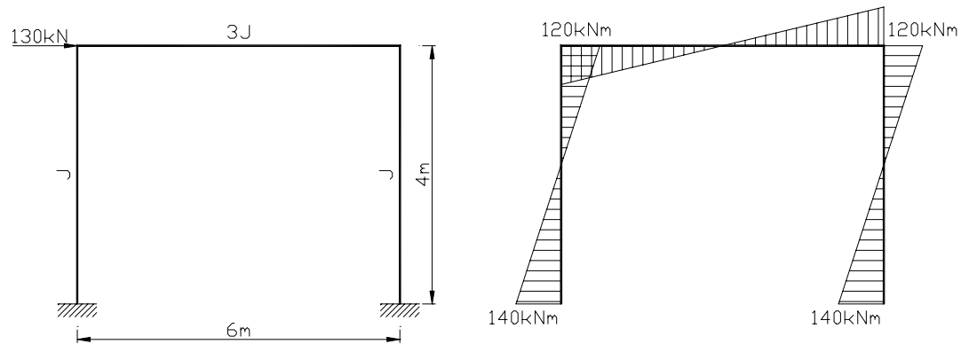
Hình 8. Sơ đồ lực và kết quả nội lực theo giải tích [5]
